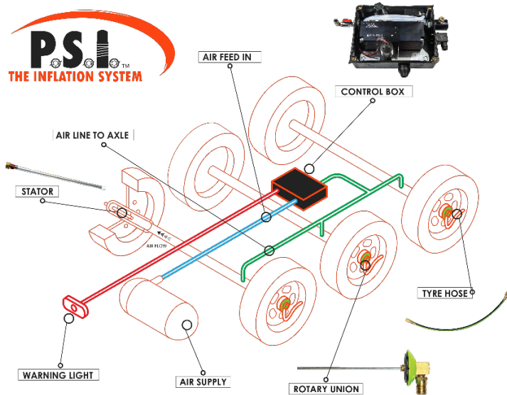
Schéma 1: Constitution du Système
