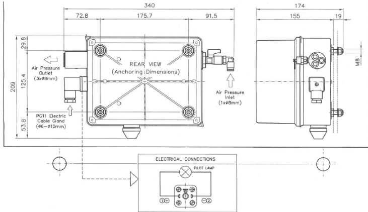
Schéma 2: Boite de Contrôle
